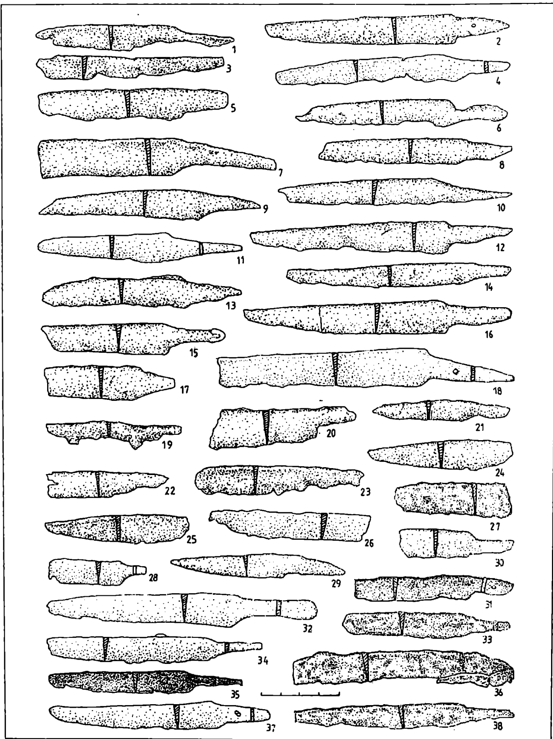
Fig. 28 Cuțite din fier.
