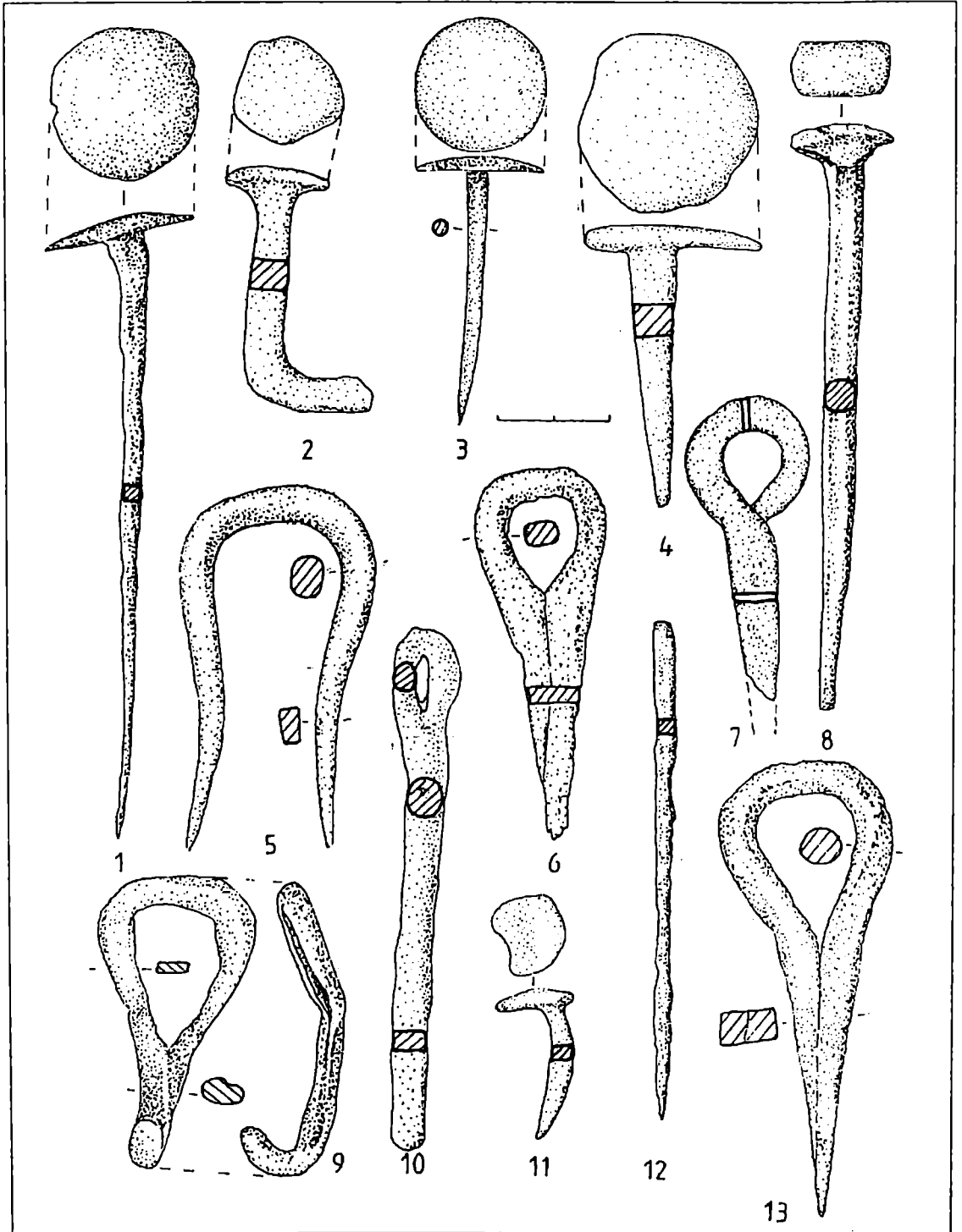
Fig. 44 Piroane (1-2, 4, 8), cuie (3, 11), împungător(12), fățâni (6, 9, 13), scoabă (5), încuietoare (7) și bară (10) din fier și bronz (3).
