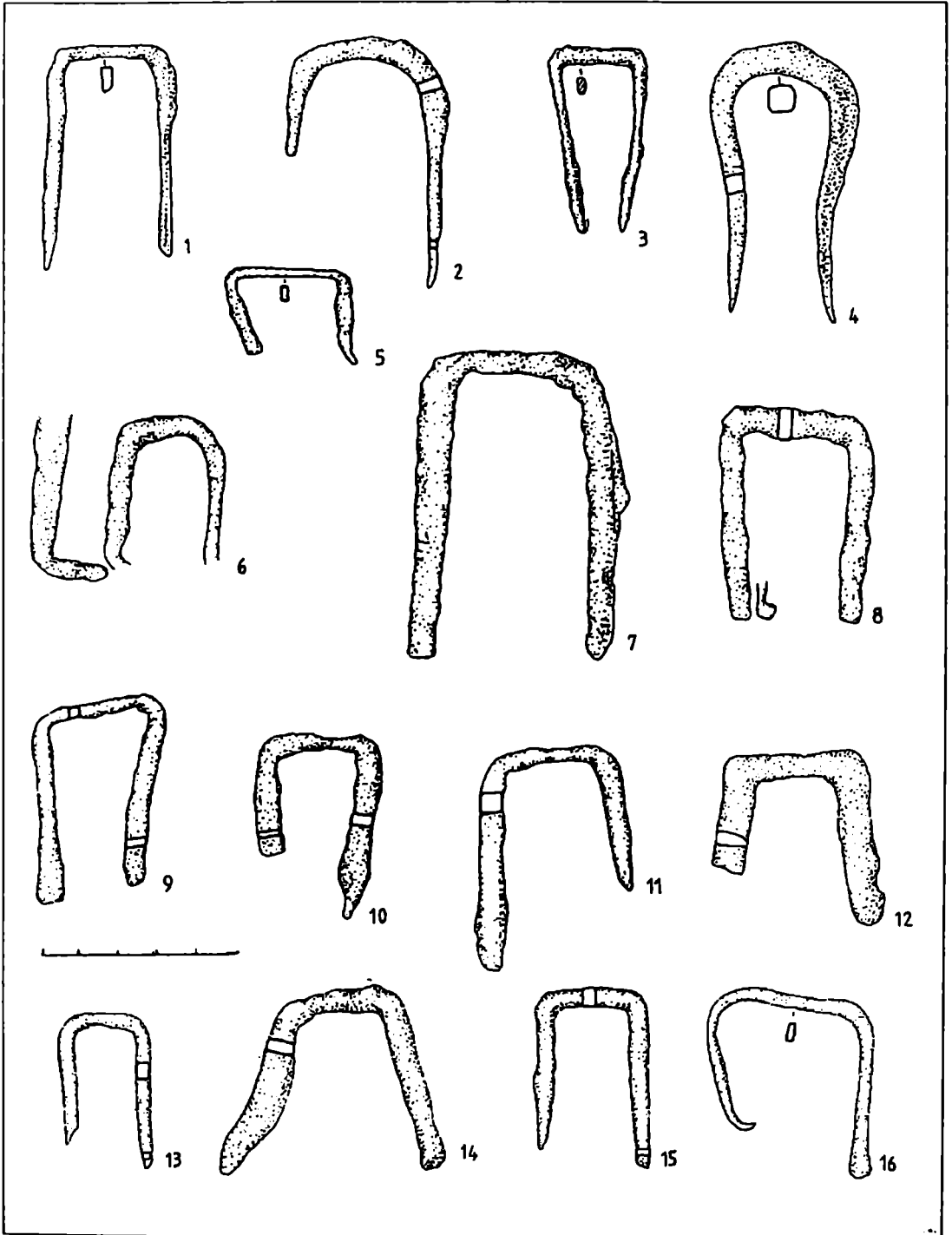
Fig. 49 Scoabe din fier.
