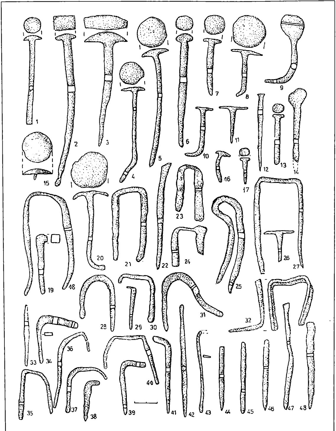
Fig. 48 Cuie (1-2, 4-11, 15-16, 20, 26), piron (3), dornuri (12-14, 17), scoabe (18-19, 21-25, 27-32, 34-41, 48) și împungători din fier.
