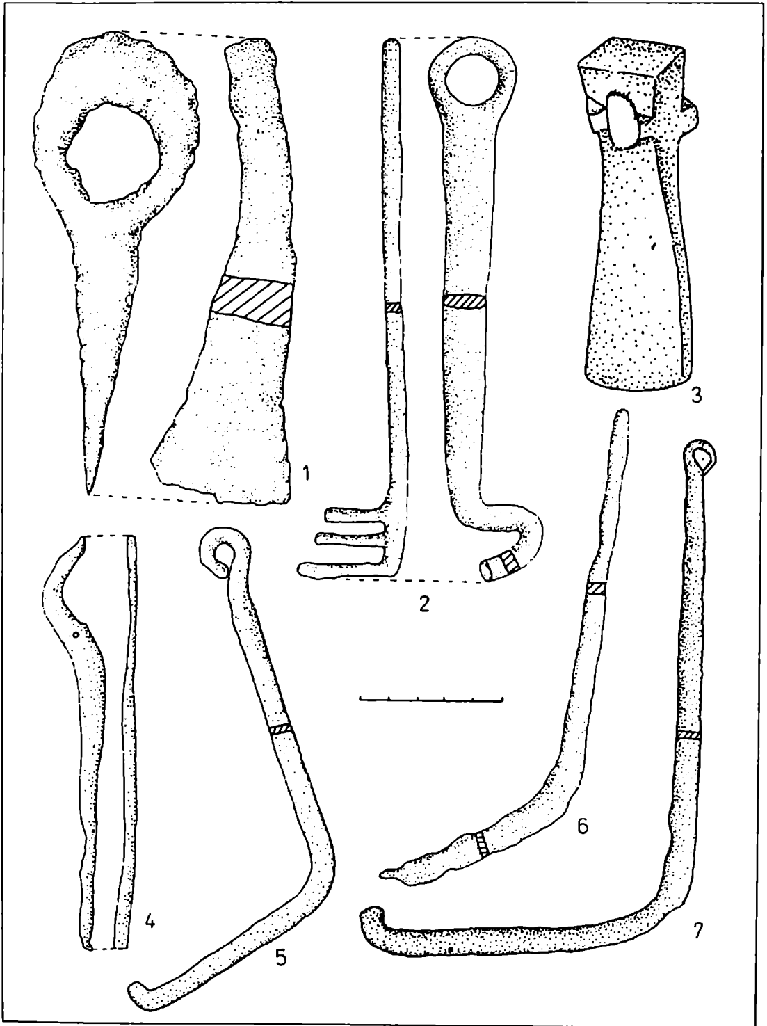
Fig. 21. Topor (1), teslă (3), clește (4) și chei (2, 5-7) de fier.
