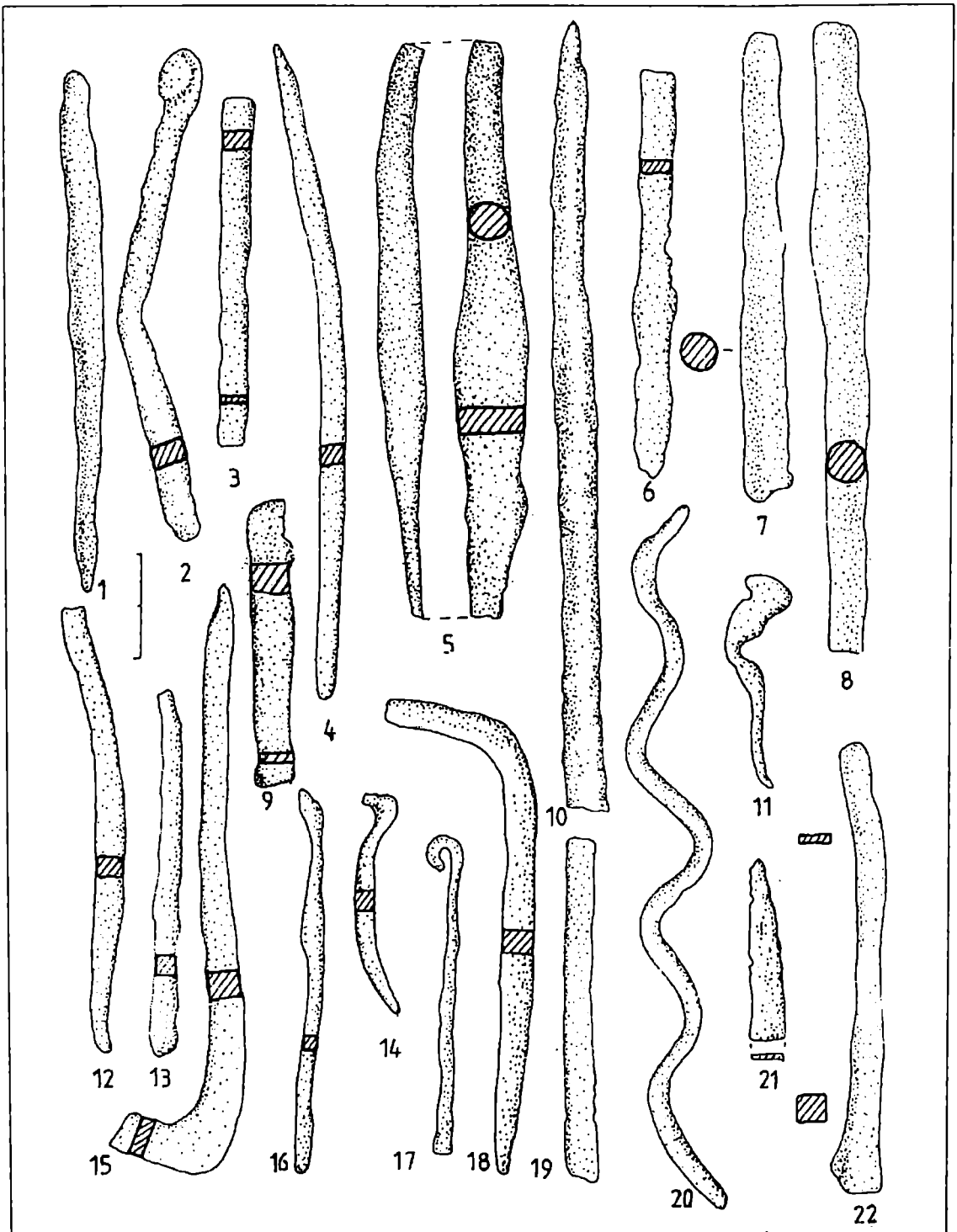
Fig. 36 Bare (1-2, 6-10, 12-13, 16, 18-19, 22), daltă (3), străpungători (4-5, 21), cui (11), cârlige (14, 17), scoabă (15) și sârmă (20) din fier.
