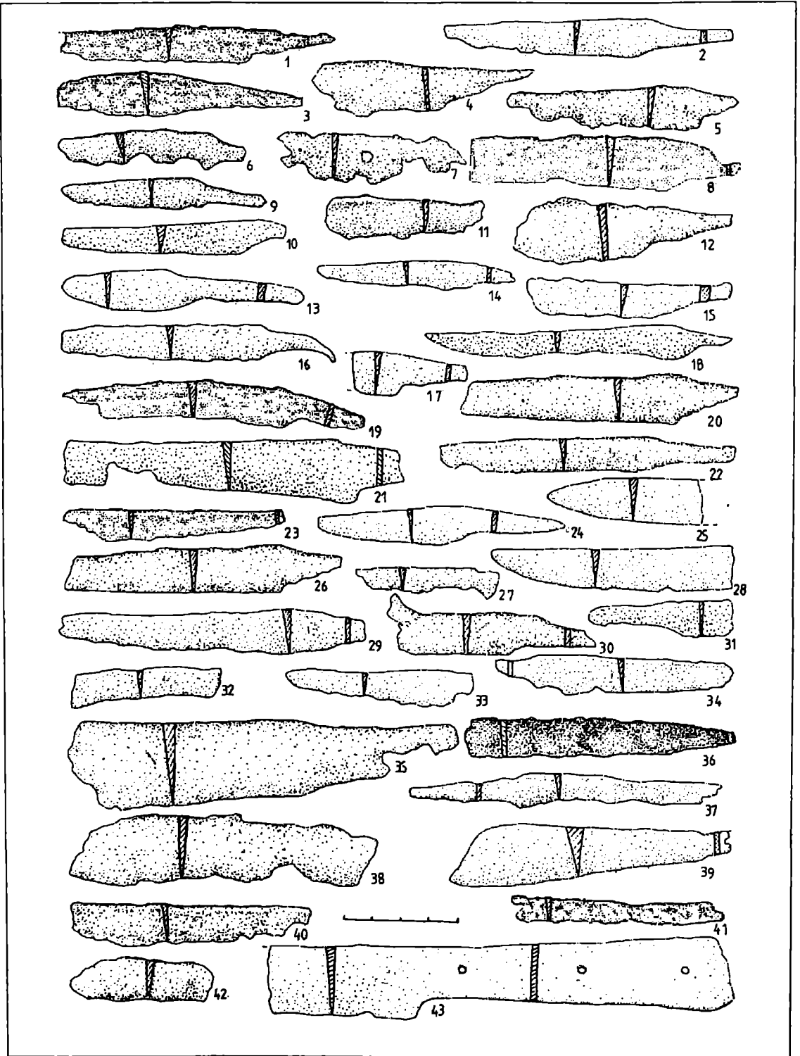
Fig. 30 Cuțite din fier.
