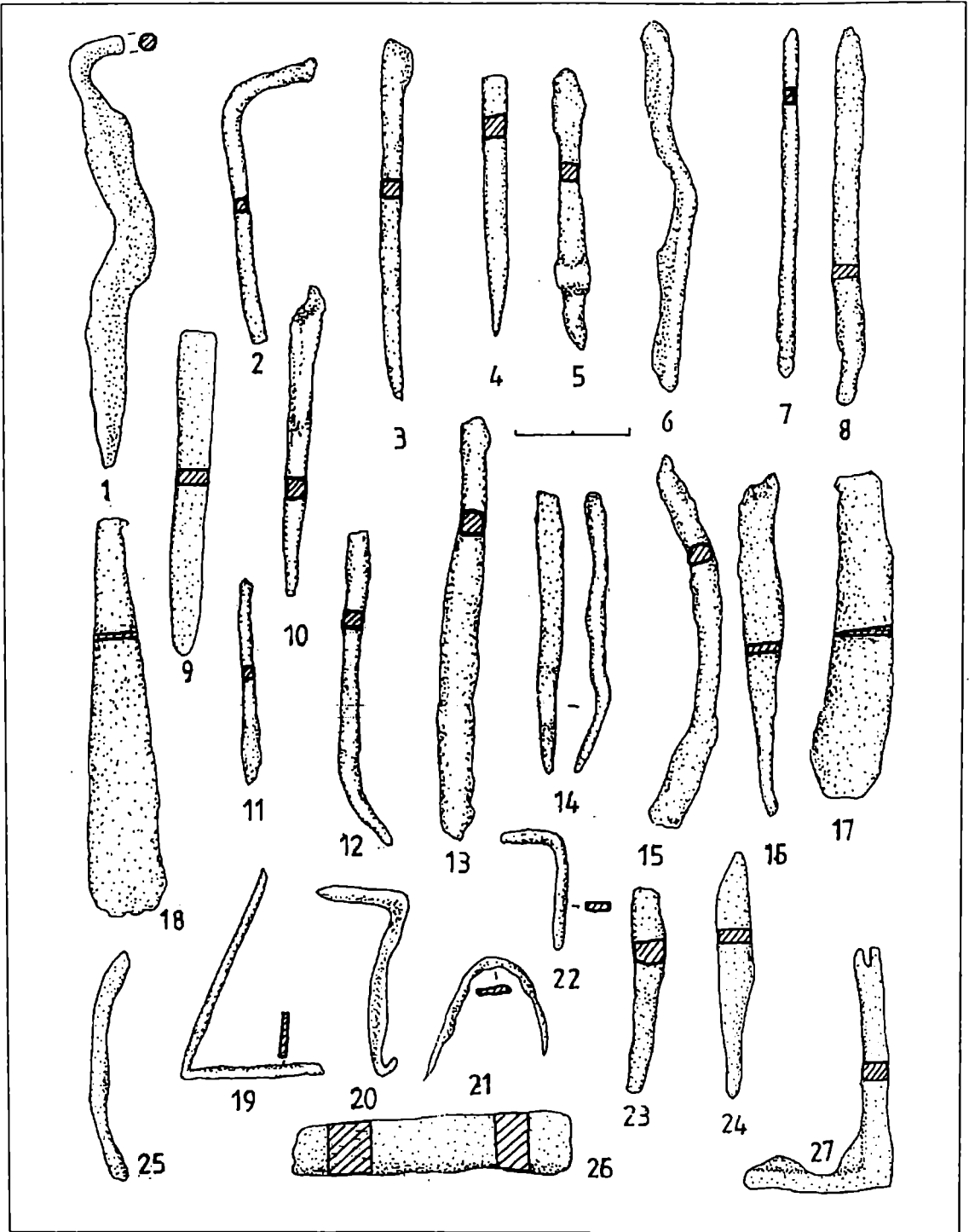
Fig. 38 Scoabe (1-2, 4, 10-12, 14, 19, 22, 24-25), străpungători (3, 23), cui (11), pilă (16), cuțit (17), daltă (9), fragmente de tablă (18, 20-21) și diferite bare (5-8, 13, 15, 27) din fier.
