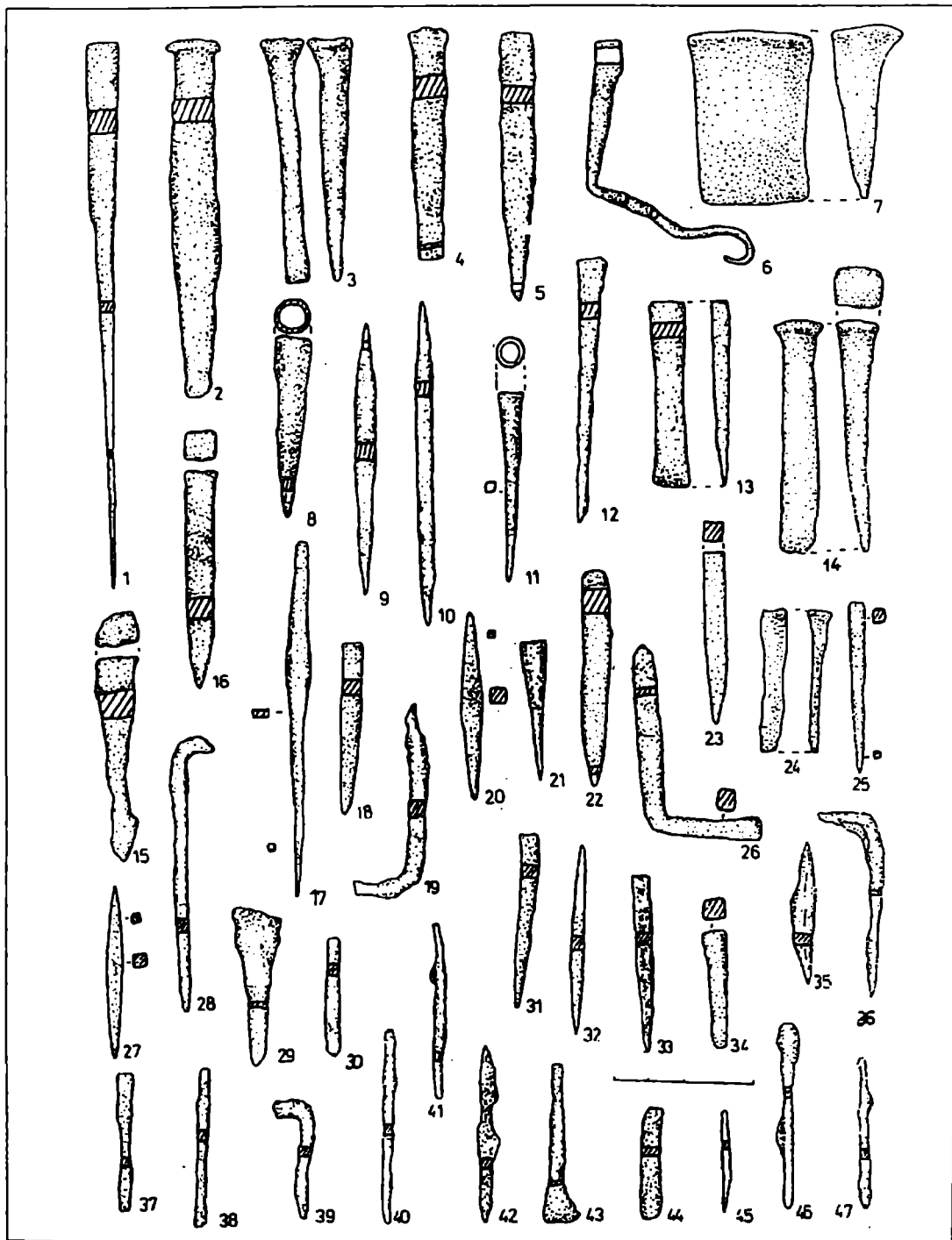
Fig. 35 Dornuri (2, 5, 15-16, 22, 25, 34), străpungători (1, 6, 8-12, 17-18, 20-21, 23, 27-29, 31-33, 35, 40-42, 45), dălți (3-4, 13-14, 24, 43), nicovală (7), scoabe (19, 26, 36-37, 39), cui (30) și bare (38, 44, 46-47) din fier.
