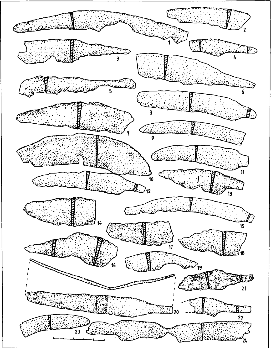
Fig. 26 Seceri (1-2, 9, 15, 23), cosoare (4-8, 10-13, 16, 19, 21-22), pilă (20) și cuțite (3, 14, 17-18, 24) din fier.
