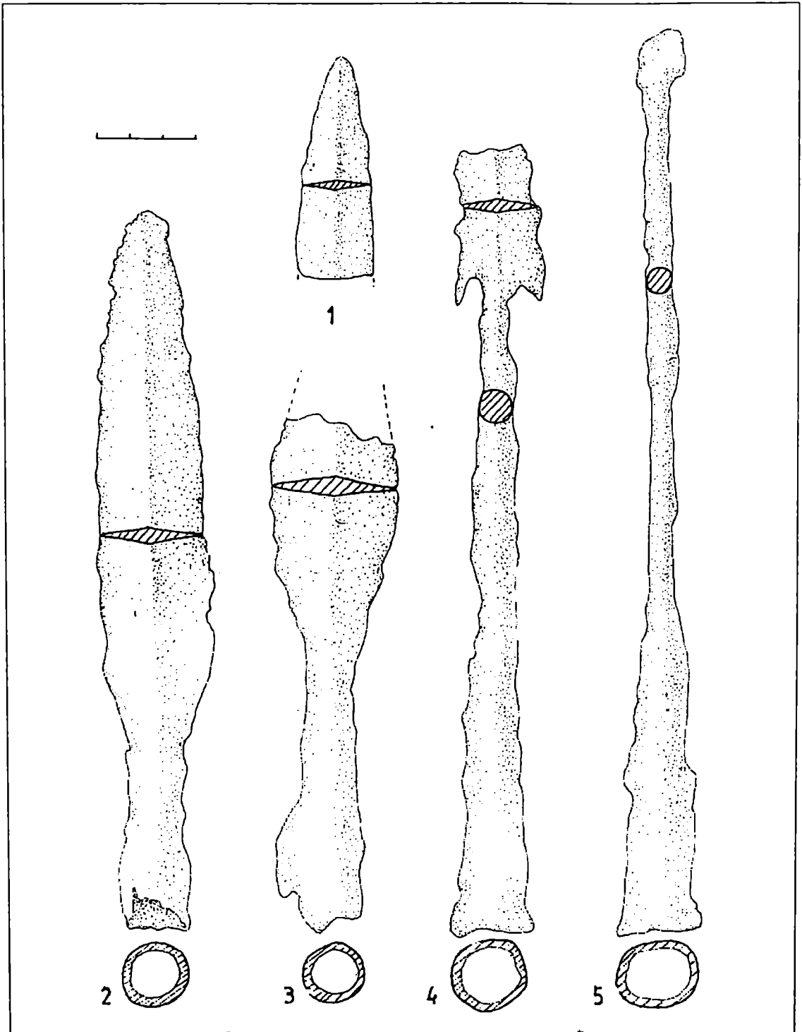
Fig. 54 Vârful de lance din fier.
