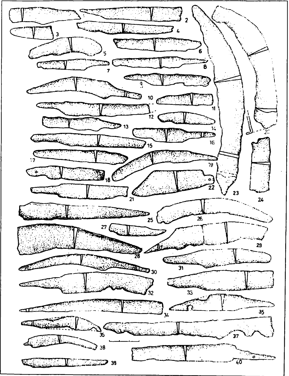
Fig. 27 Cuțite (1-9, 11-13, 15-18, 21-22, 24-25, 27, 32-35, 37, 39-40), cosoare (10, 14, 19, 29-31, 36, 38) și seceri (20, 23, 26, 28) din fier.
